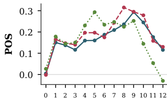
Base GPT-2
